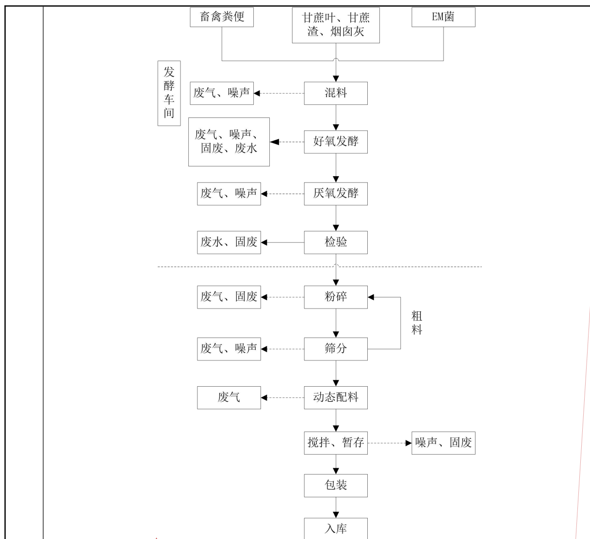
图 2-2 项目生产工艺流程及产污节点图
