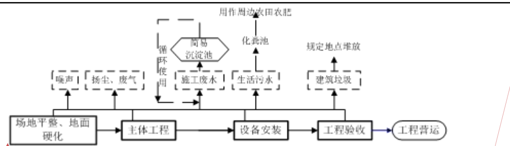
图 2-1 施工期工艺流程及产污情况
