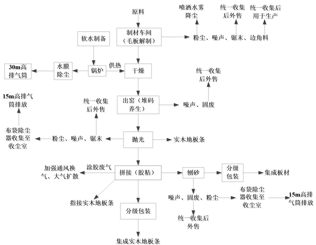
图 2-3 本项目生产加工工艺流程图及产污环节示意图
