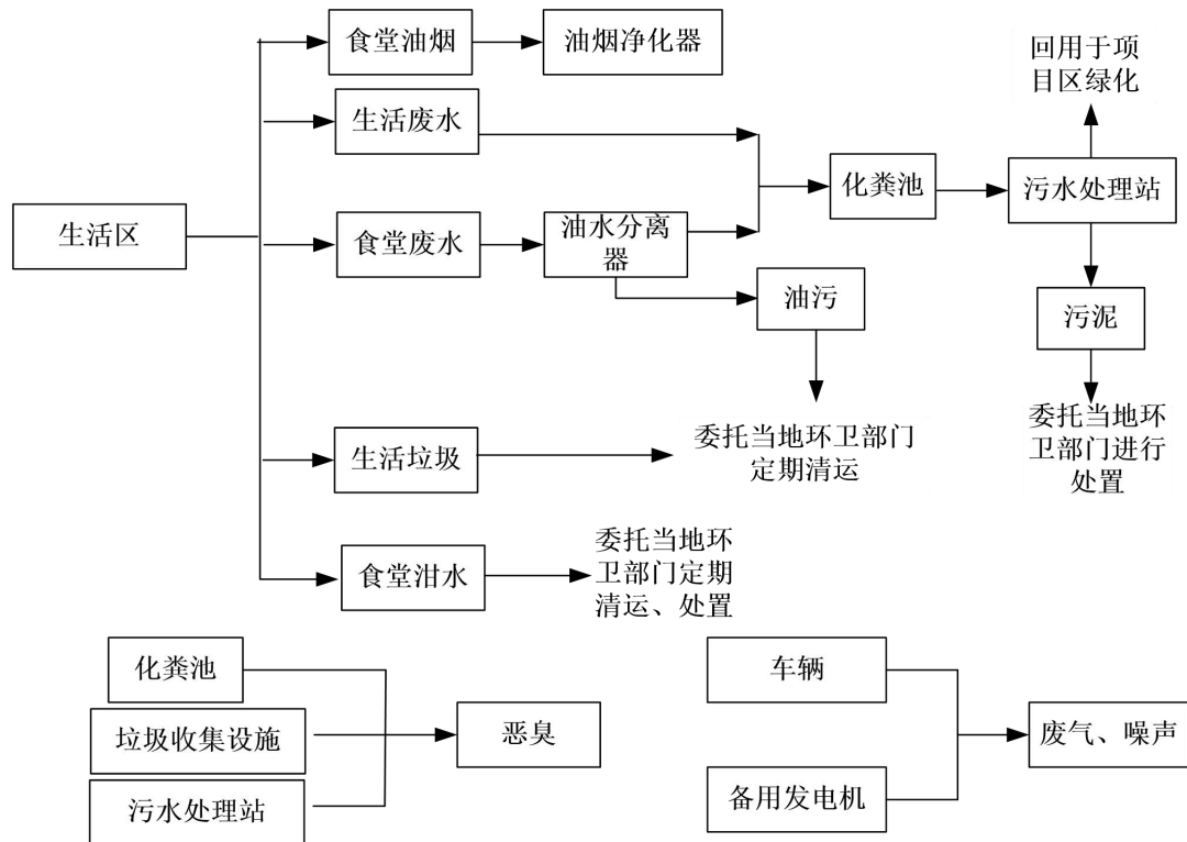
图 2-5 营运期厂区日常运行产污环节分析图
